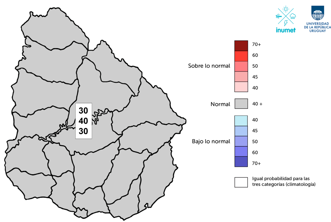
FIGURA 7 Probabilidades en porcentajes de los terciles de temperatura. Meses: diciembre - enero - febrero 2026 - 2027.
